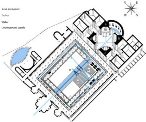
Fig. 41 - The irrigation plan of the Piazza d'Oro
